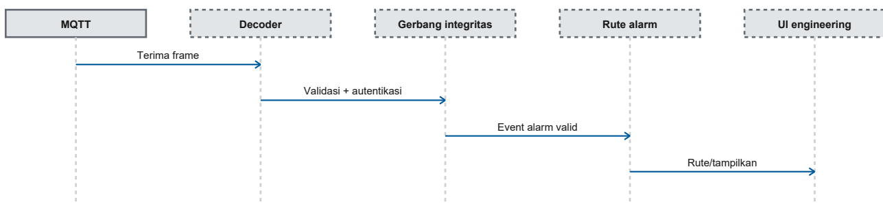
Gambar 4. Alarm routing pada Server.
